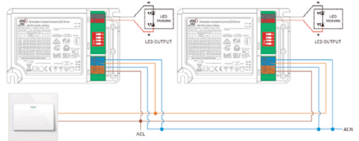
Esquema de conexión. Schéma de connexion PUSH
