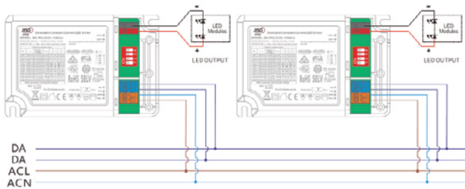
Esquema de conexión. Schéma de connexion DALI
